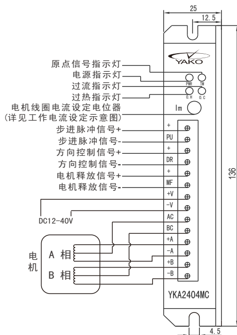
驱动器接线示意图
