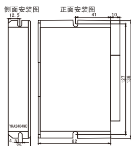
采用侧面安装，散热效果较好
